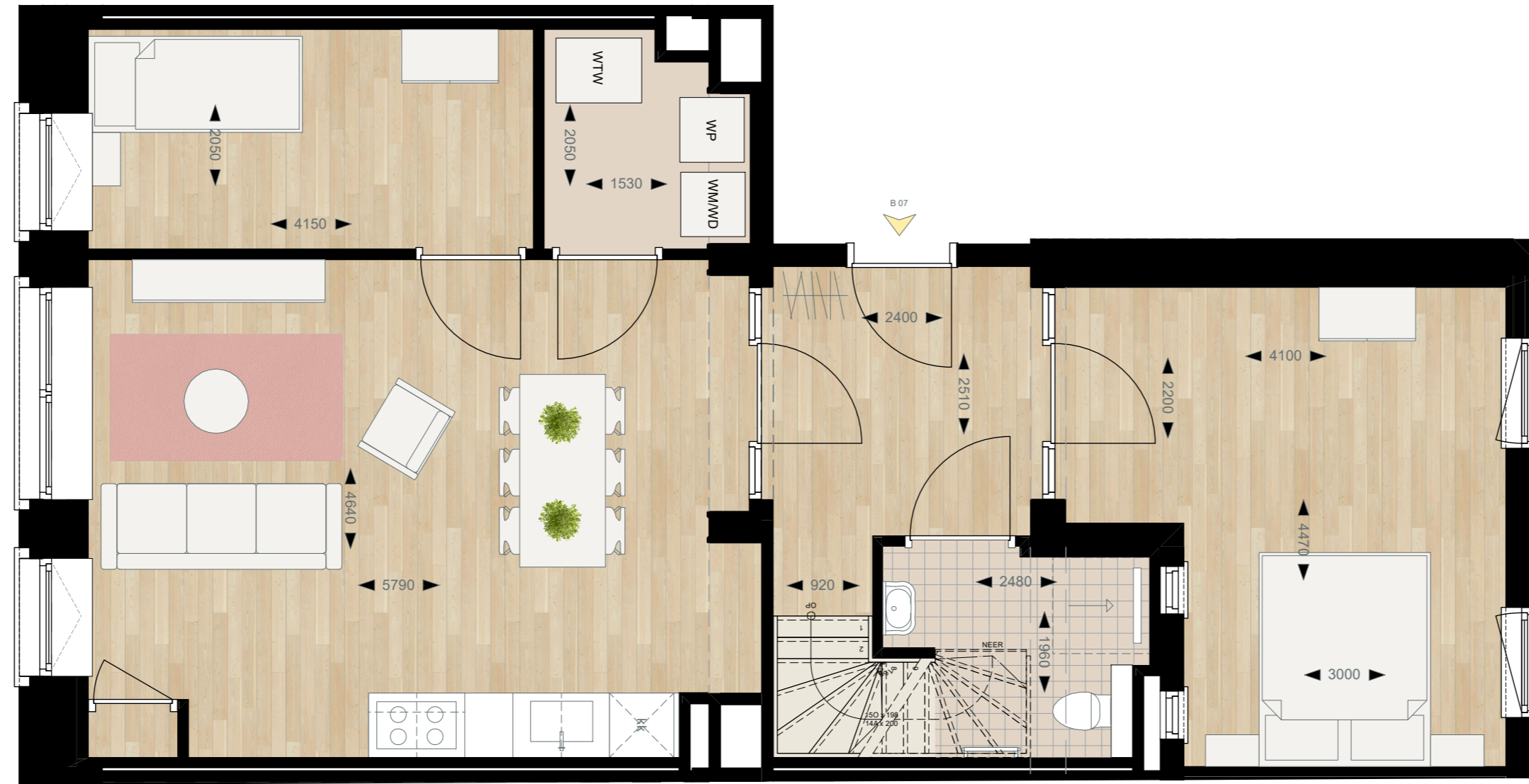
eerste verdieping - schaal 1:50
